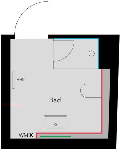
Grundriss Bad, Maßstab ca. 1:50
