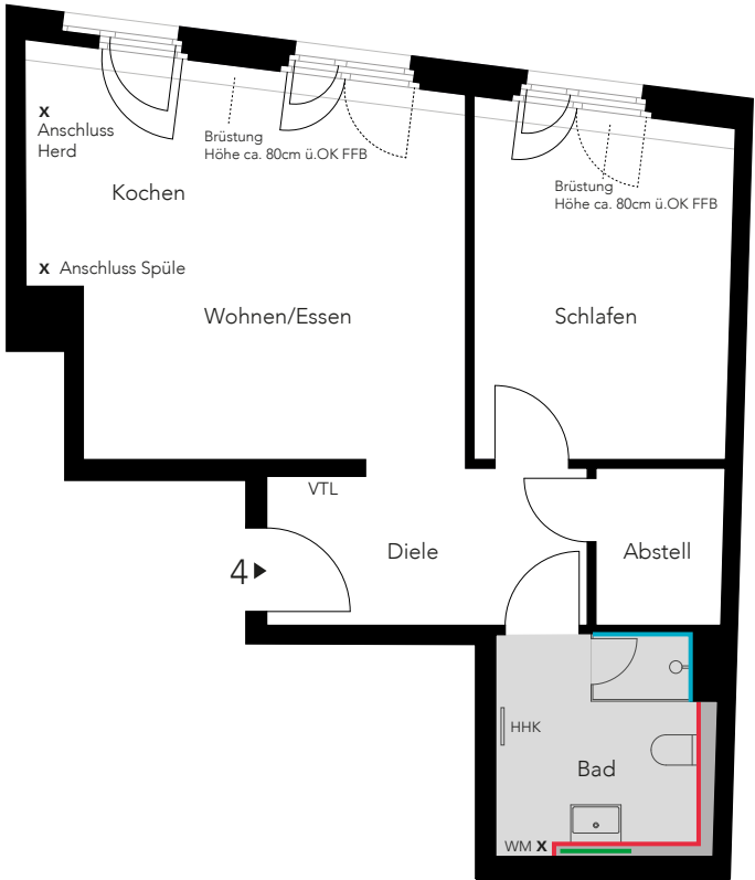
Wohnungsgrundriss Maßstab ca. 1:100
